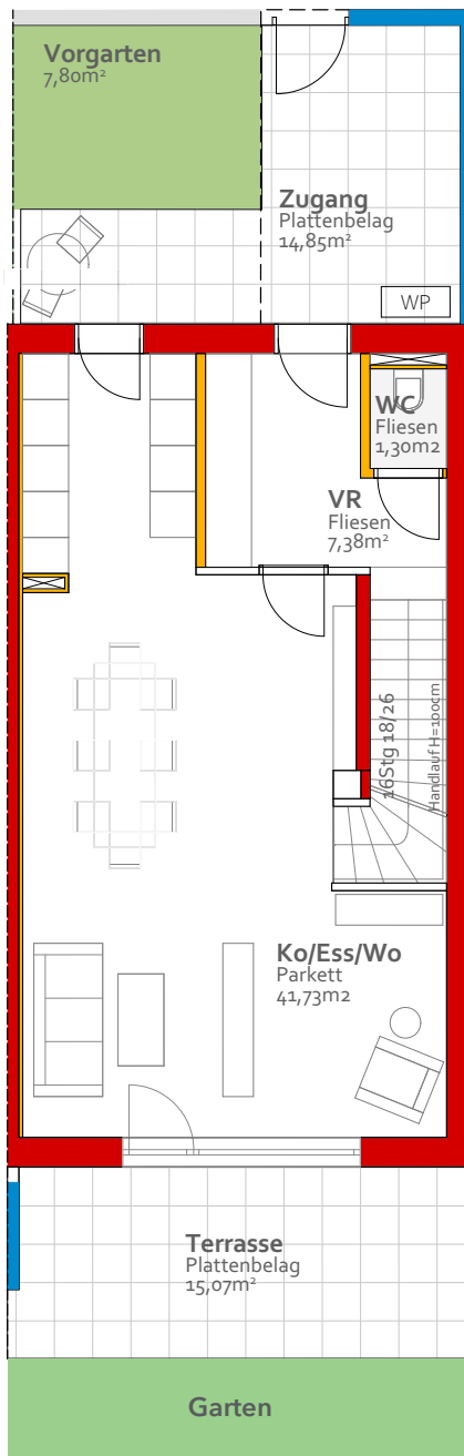
Erdgeschoss
