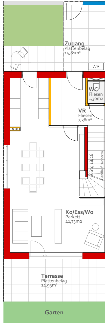
Erdgeschoss
