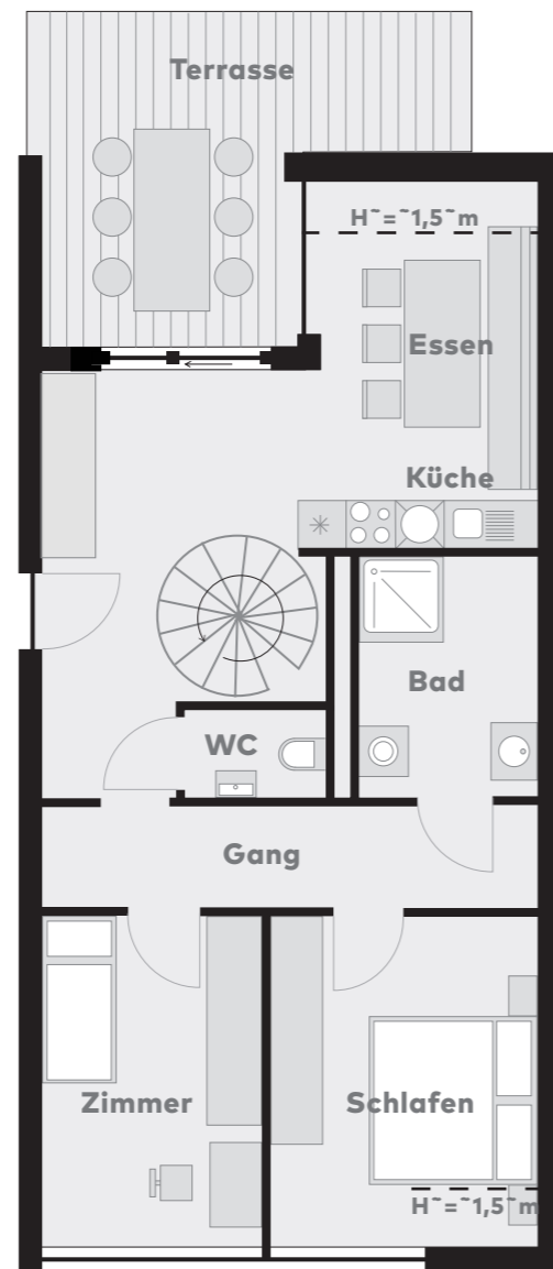
Dachgeschoss
